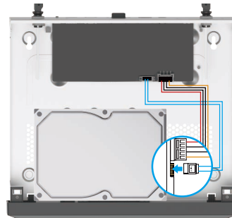
Connexion du câble de données
